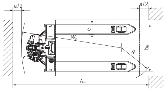
ECH 12C/15C vista de cima
