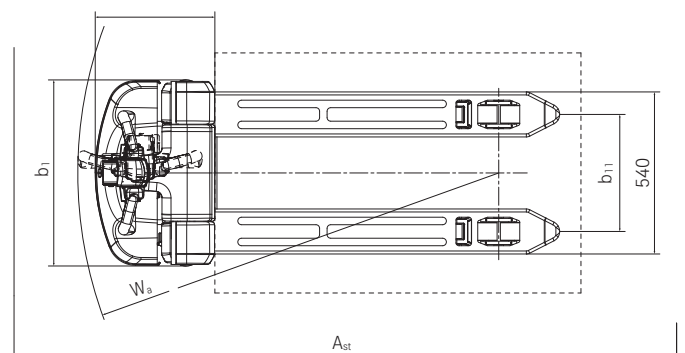
ECH 15 vista de cima
