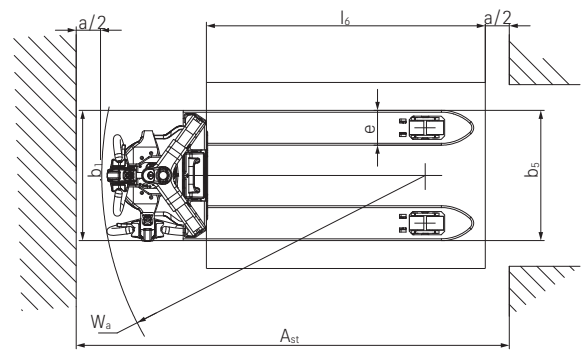
ECH 12 vista de cima
